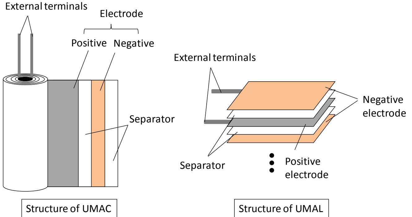
Fig.5: Structure of UMA series
