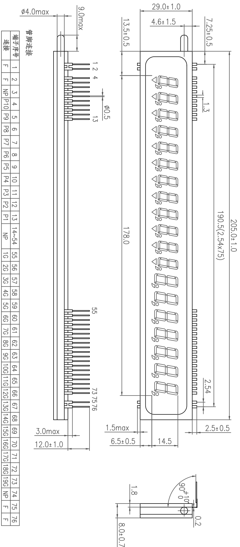
外形图
